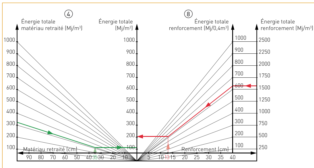
Figure 29 : diagramme de comparaison environnementale (Energie)
