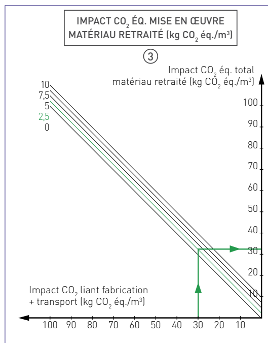
Figure 33 : zone Retraitement - Quadrant impact CO 2 mise en œuvre
