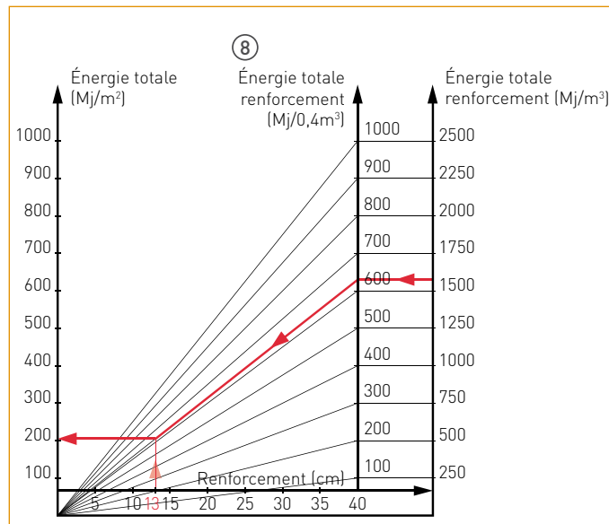
Figure 28 : zone renforcement - Quadrant Energie totale (Mj/m 3 et MJ/m 2 )
