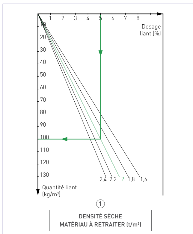
Figure 30 : zone Retraitement - Quadrant densité sèche matériaux.
