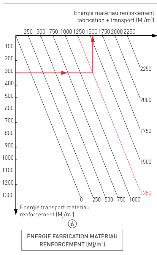
Figure 26 : zone renforcement - Quadrant Energie extraction et fabrication matériaux
