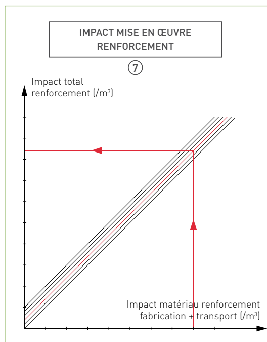
Figure 8 : zone renforcement - Quadrant impact mise en oeuvre matériau
