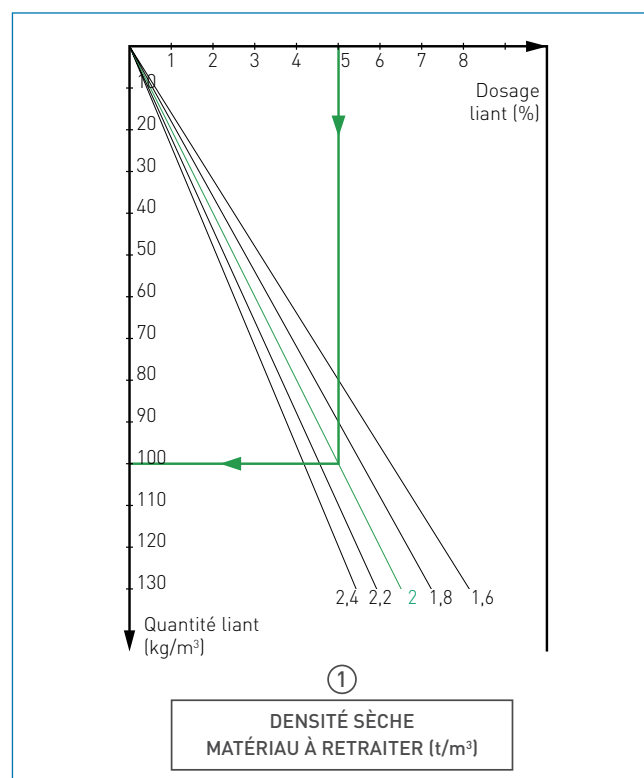
Figure 11 : zone matériau retraité - Quadrant densité sèche matériau
