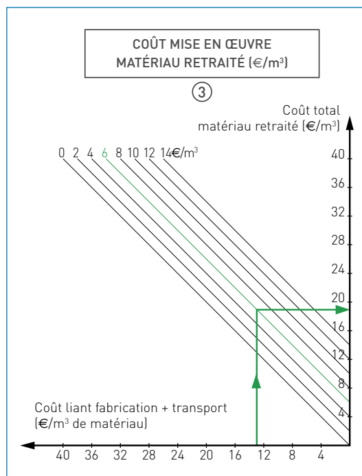
Figure 13 : zone matériau retraité - Quadrant coût mise en oeuvre
