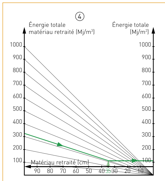
Figure 24 : zone matériau retraité - Quadrant Energie totale (Mj/m 3 et MJ/m 2 )
