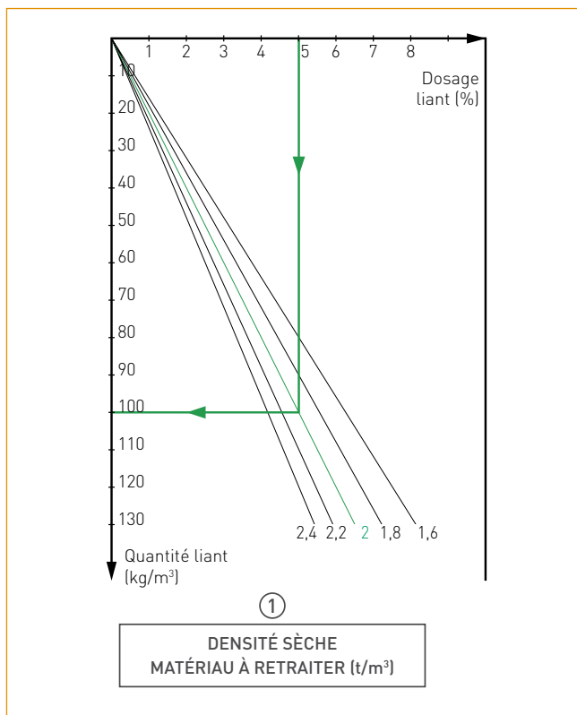
Figure 20 : zone retraitement - Quadrant densité sèche matériau
