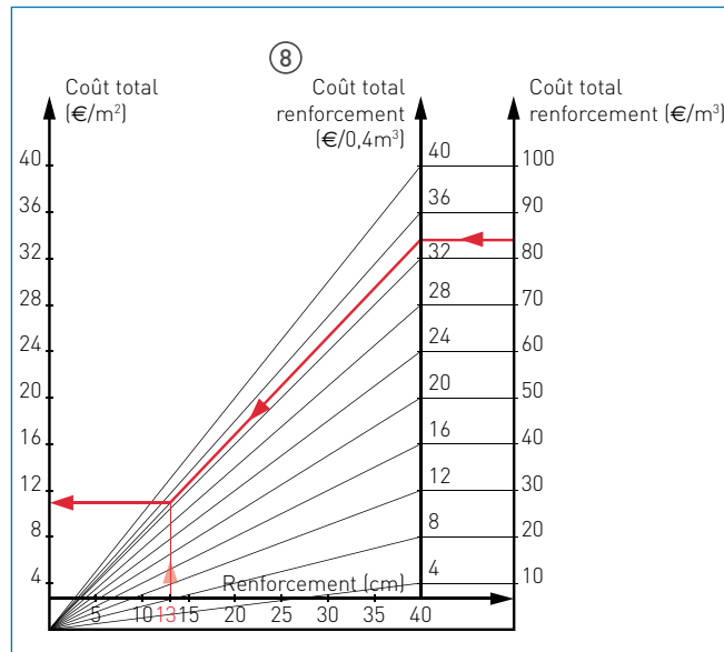
Figure 18 : zone renforcement - Quadrant coût total (€/m 2 et €/m 3 )
