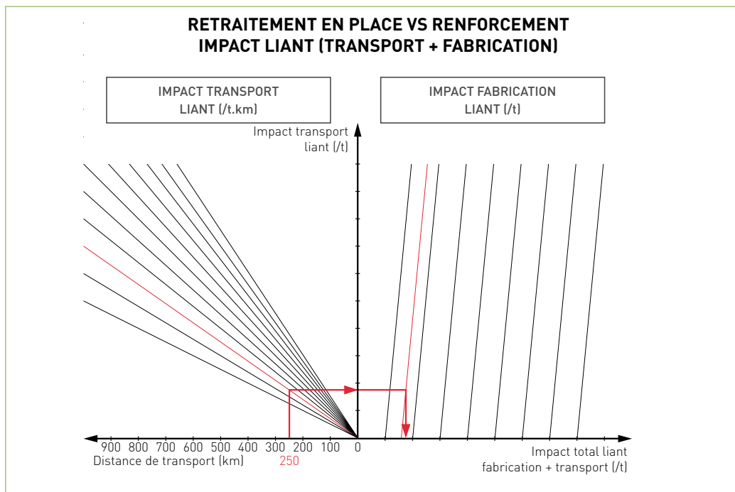
Figure 3 : diagramme d'évaluation de l'impact du liant (fabrication + transport)
