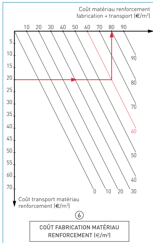
Figure 16 : zone renforcement - Quadrant coût extraction et fabrication matériaux
