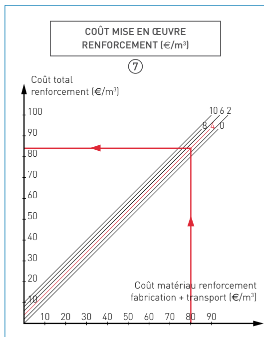
Figure 17 : zone renforcement - Quadrant coût mise en oeuvre matériaux
