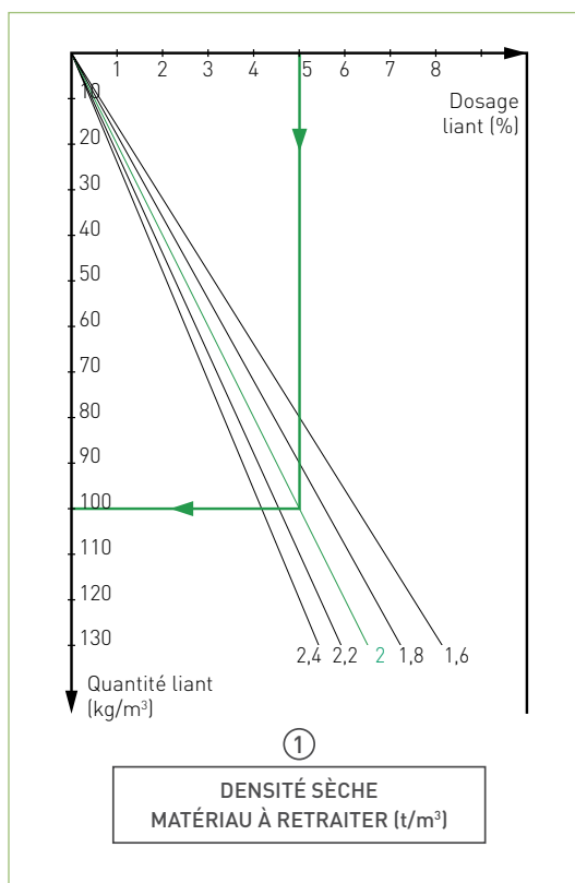
Figure 1 : zone matériau retraité - Quadrant densité sèche matériau
