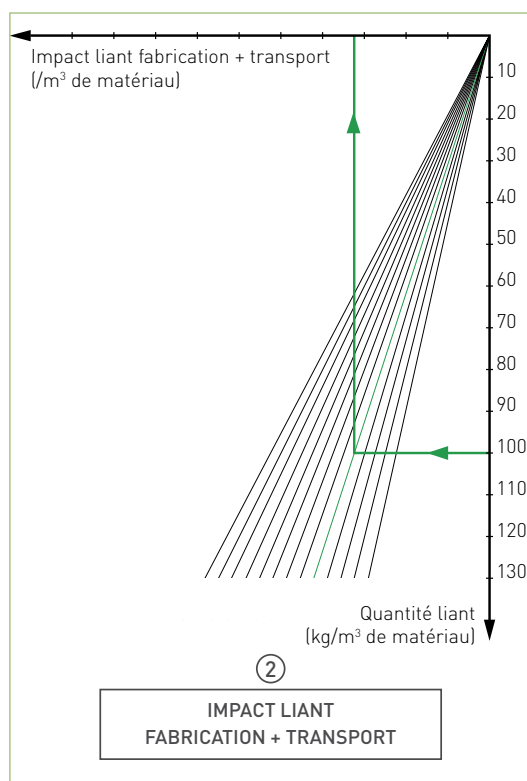
Figure 2 : zone matériau retraité - Quadrant impact liant
