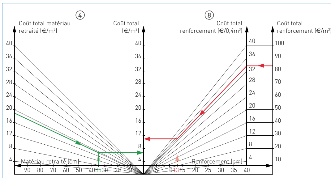
Figure 19 : diagramme de comparaison des coûts.
