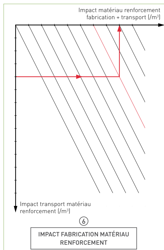
Figure 7 : zone renforcement - Quadrant impact extraction, transport des constituants et fabrication matériau
