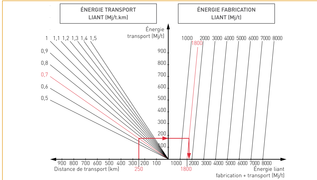
Figure 22 : diagramme d'évaluation de l'Énergie du liant (fabrication + transport)
