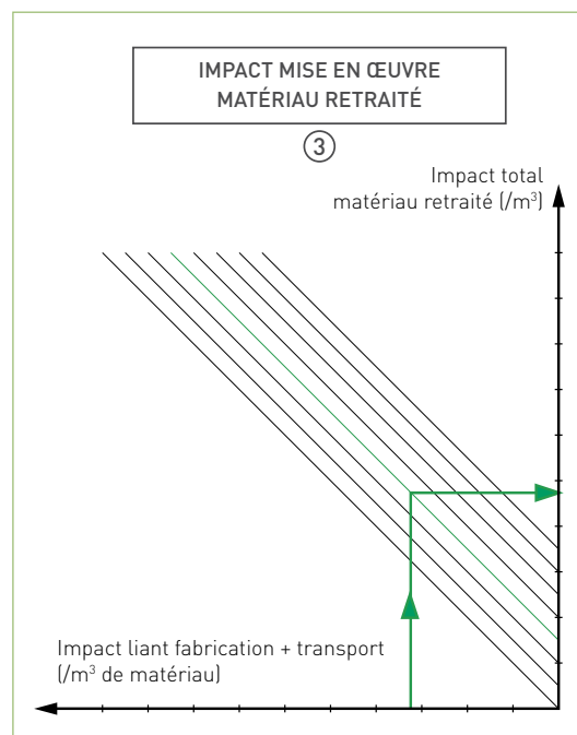
Figure 4 : zone matériau retraité - Quadrant impact mise en oeuvre
