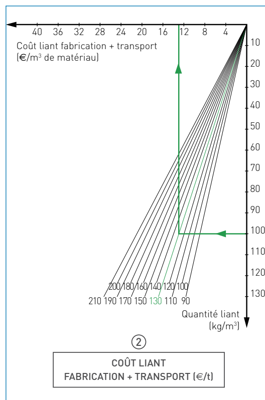
Figure 12 : zone matériau retraité - Quadrant coût liant
