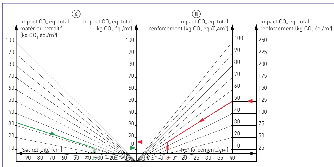
Figure 42 : diagramme de comparaison environnementale (impact CO 2 )
