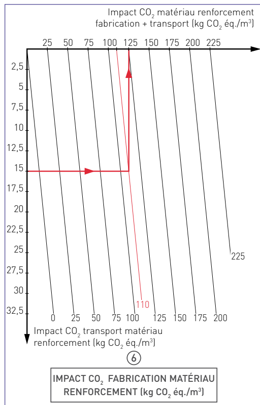
Figure 36 : zone renforcement - Quadrant impact CO 2 extraction et fabrication matériau
