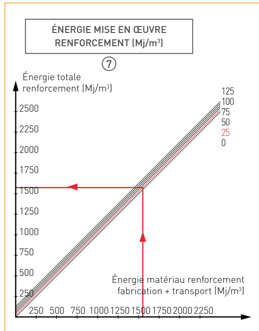
Figure 27 : zone renforcement - Quadrant Energie mise en oeuvre matériaux
