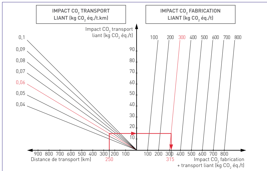
Figure 32 : diagramme d'évaluation de l'impact CO 2 du liant (fabrication + transport)
