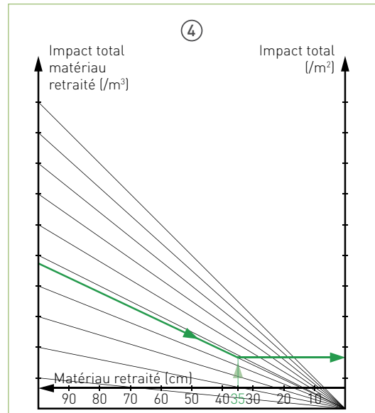
Figure 5 : zone matériau retraité - Quadrant impact total (/m³ et /m²)
