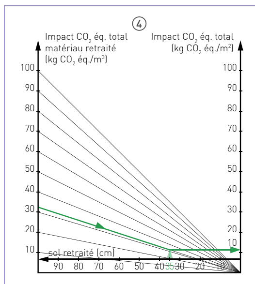
Figure 34 : zone retraitement - Quadrant impact total CO 2 (kg CO 2 éq./m 3 et kg CO 2 éq./m 2 )
