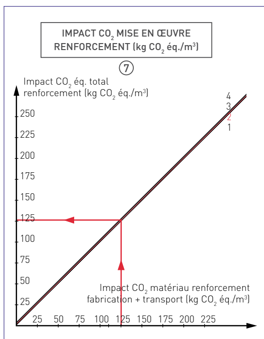
Figure 37 : zone renforcement - Quadrant impact CO 2 mise en oeuvre matériaux
