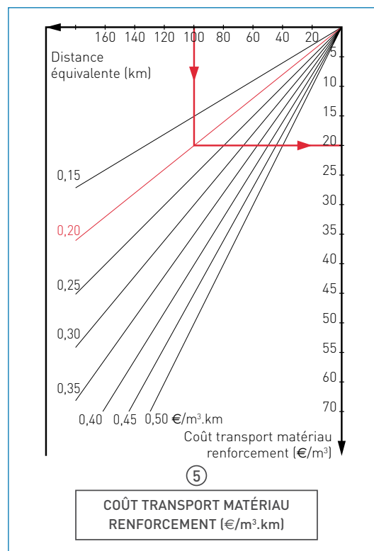
Figure 15 : zone renforcement - Quadrant coût transport matériau
