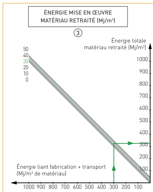
Figure 23 : zone matériau retraité - Quadrant Energie mise en œuvre
