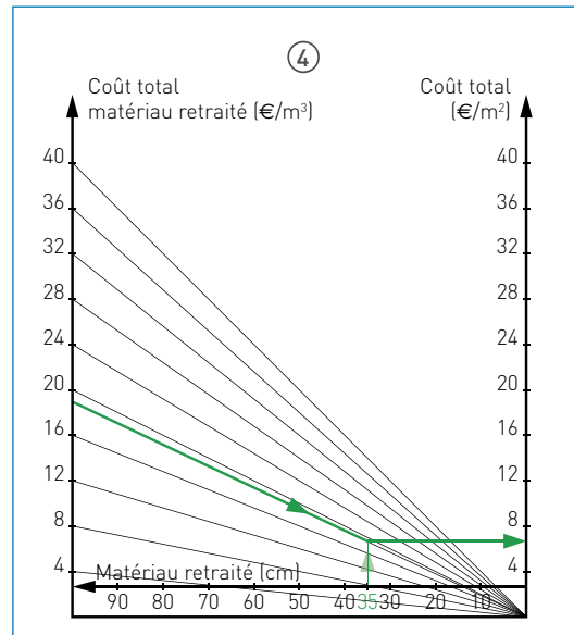
Figure 14 : zone matériau retraité - Quadrant coût total (€/m 3 et €/m 2 )
