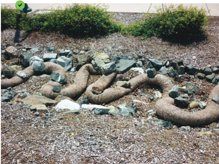
Boudin installé sur un fossé de collecte des écoulements superficiels, maintenu au sol à l'aide de blocs.
