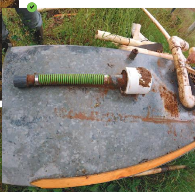
Installation d'un skimmer au sein d'un bassin de décantation provisoire.
