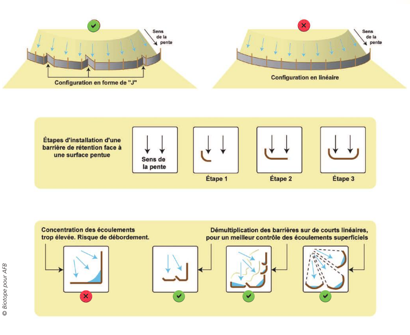
Figure 39. Principes d'installation de barrières de rétention : en série et en « J ». Source : McCullah (2007).
