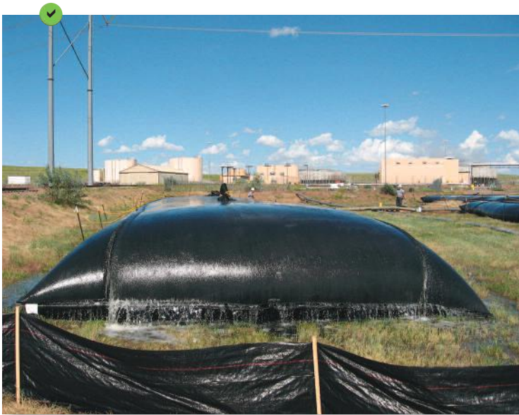
Sac à sédiments en opération.
