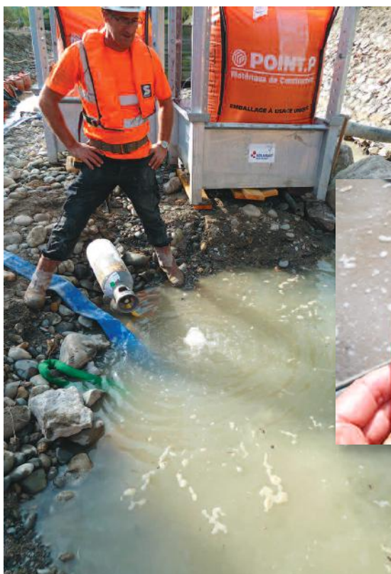
Injection de CO 2 dans une eau polluée par des laitances béton.
