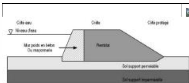
Digue composite avec soutènement par un mur poids côté rivière
