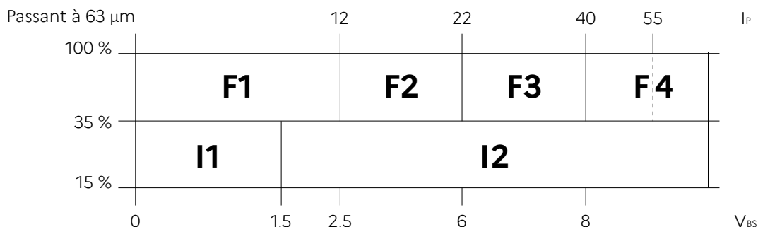
Figures 7 et 8: Synoptiques de classification des sols avec D_{\text{max}} < 63 \text{ mm}
